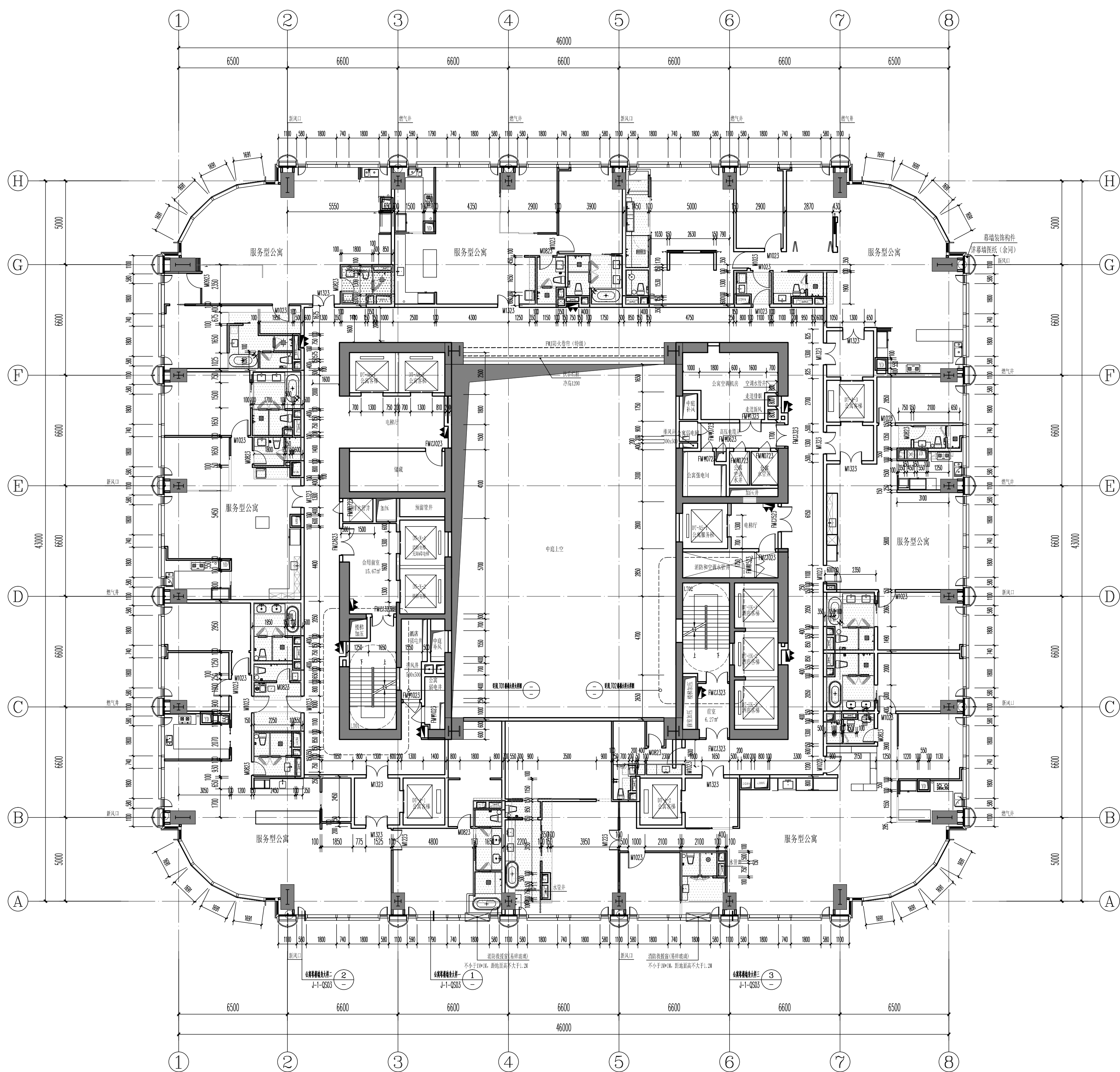
三十五~三十八层平面图 1:150
